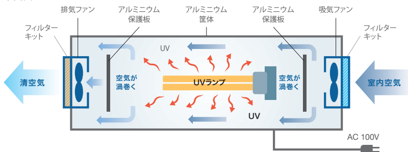
正面図
